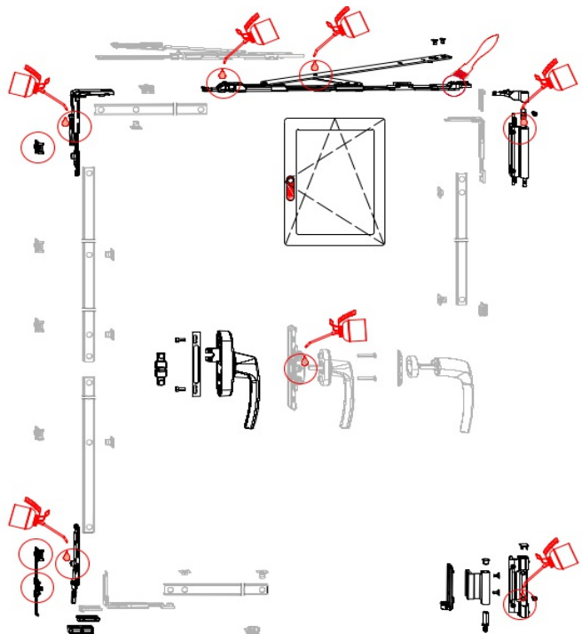
Aanbevolen smeerpunten voor draai-kiep ramen.
